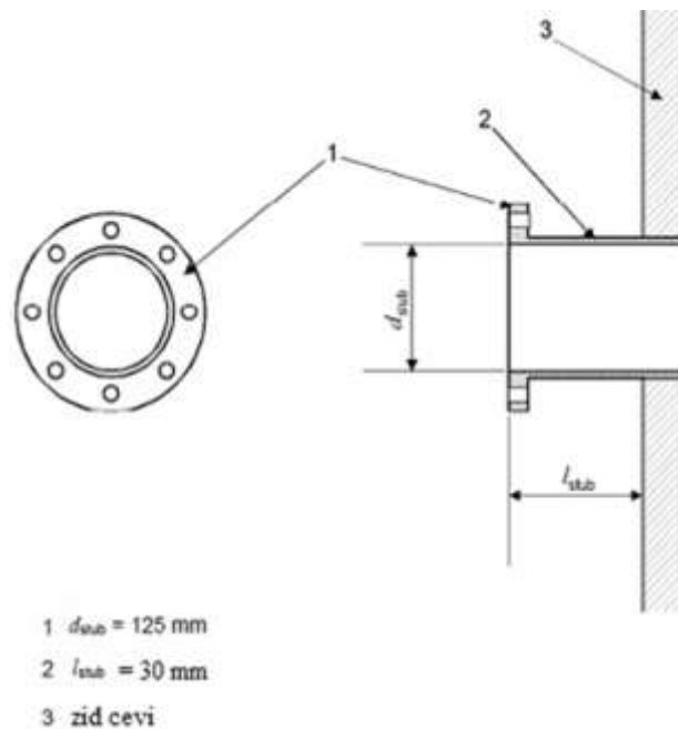
Slika A 2.1 Dimenzije i izgled otvora na mernim mestima
