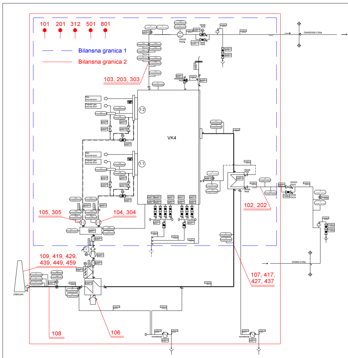
Slika 2. Šema mernih mesta na bilansnoj granici kotla
