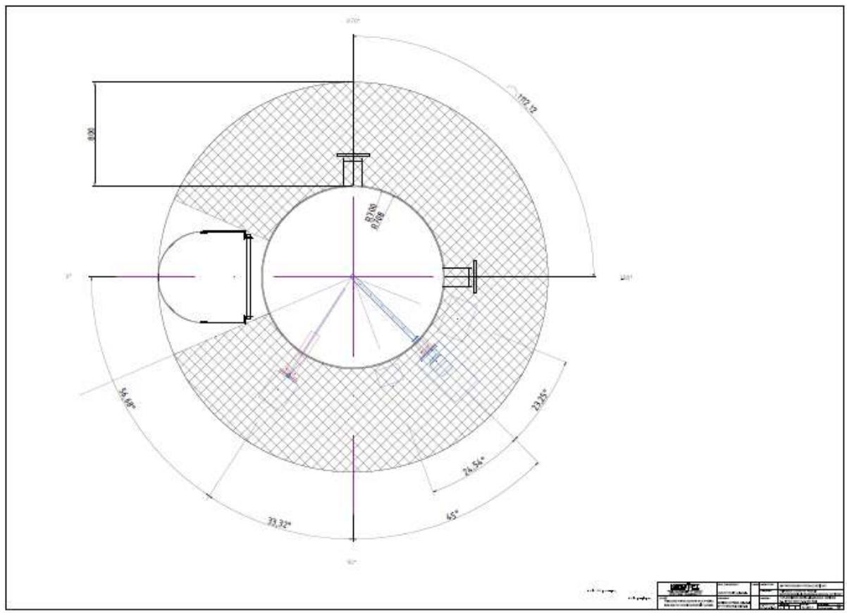
Slika A 2.7 Merno mesto za merenje emisije zagađujućih materija na dimnjaku
